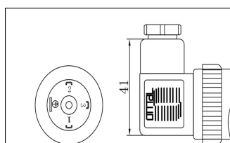
DIN43650 代码: 2D
