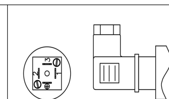
工业连接器/Industrial connector 代码1D
